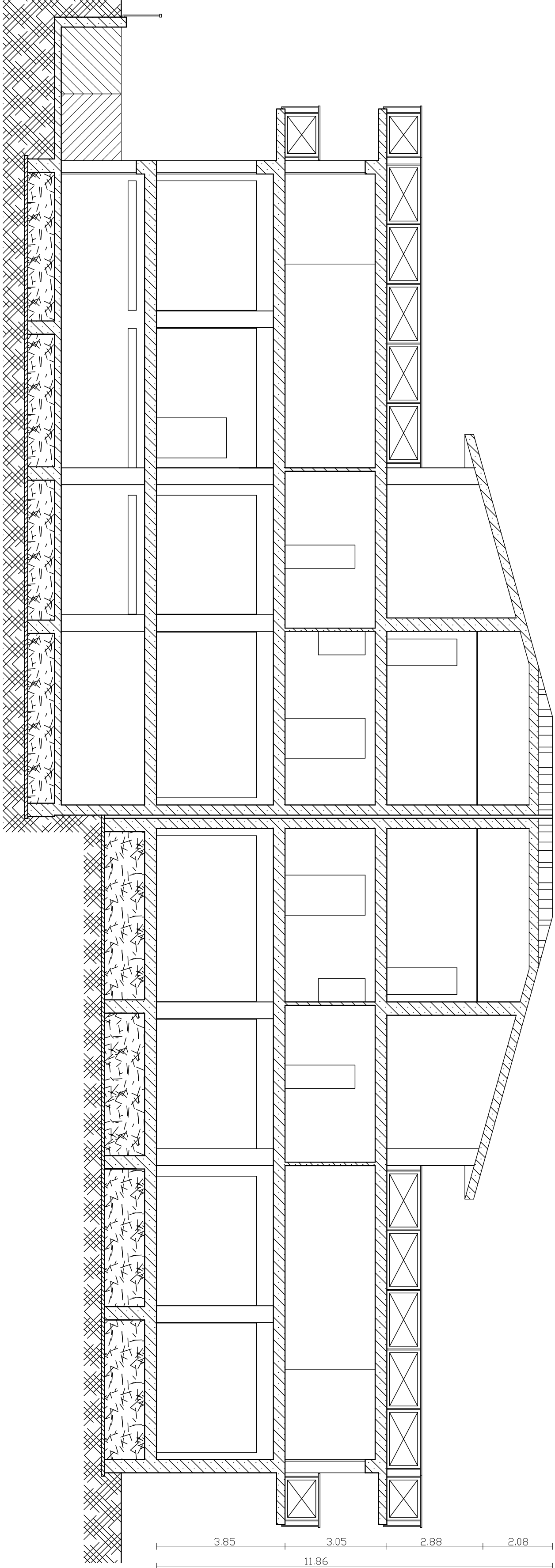
Sezione tipologia edilizia Lotto IV
