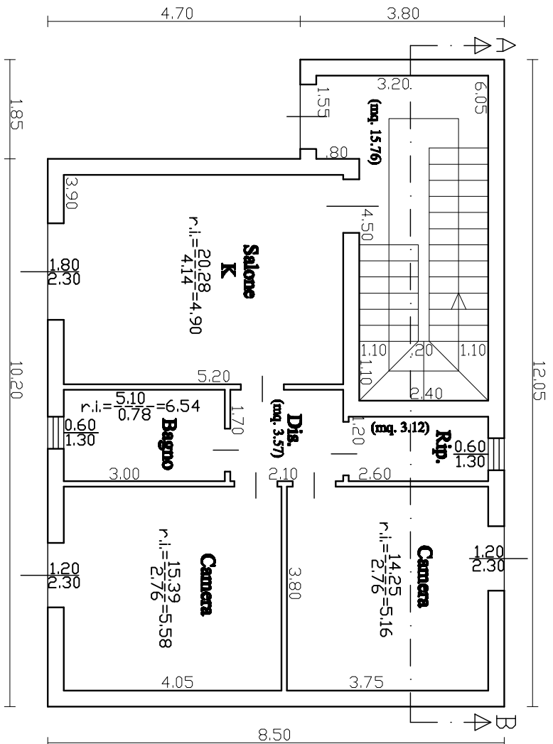
Tipologia edilizia Lotto I
