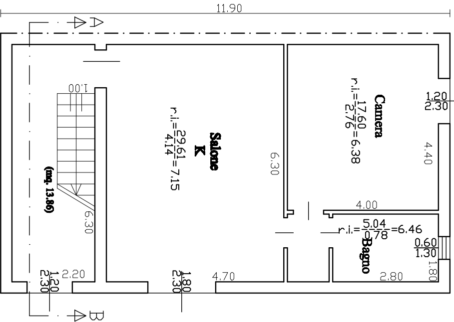
Tipologia edilizia Lotto III
