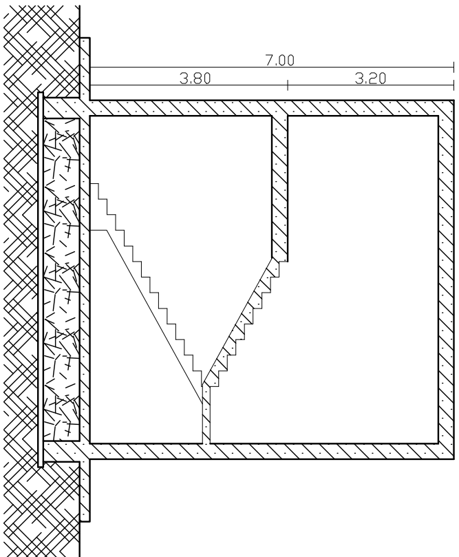
Sezione tipologia edilizia Lotto III
