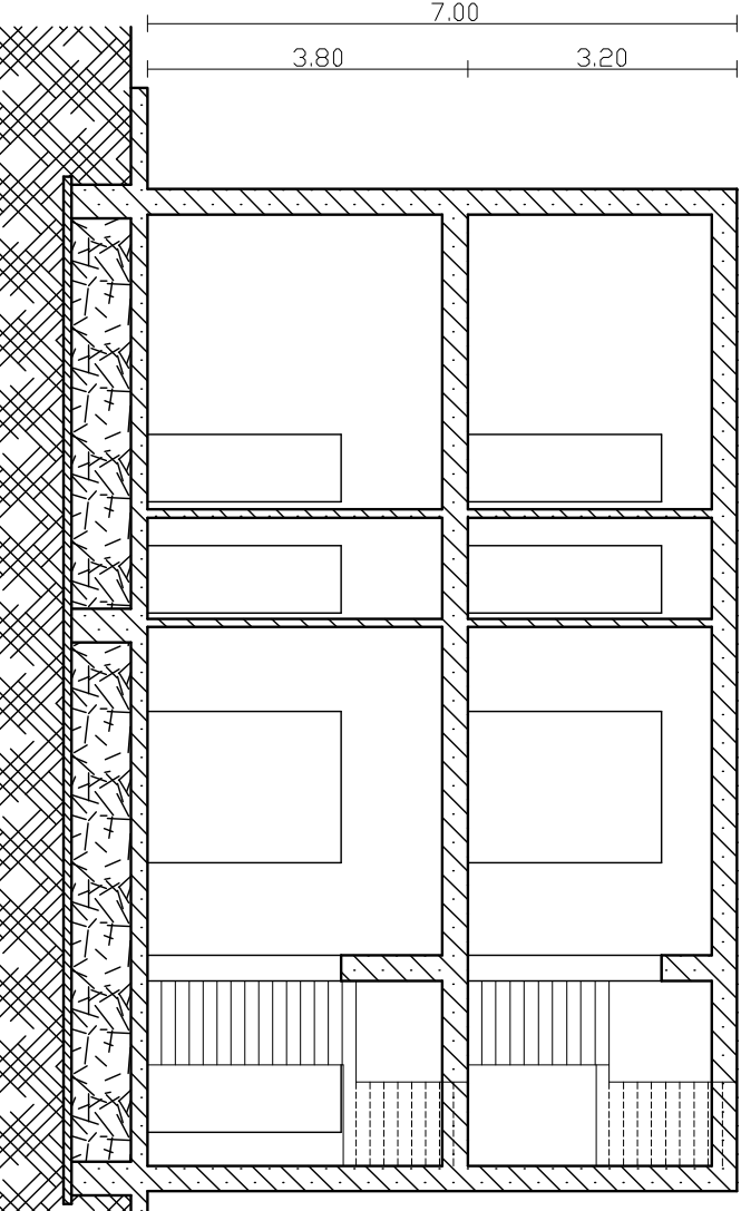
Sezione tipologia edilizia Lotto II
