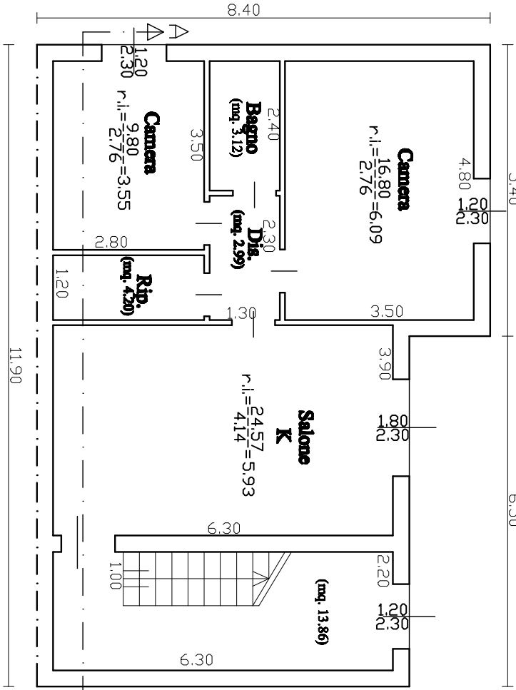
Tipologia edilizia Lotto II
