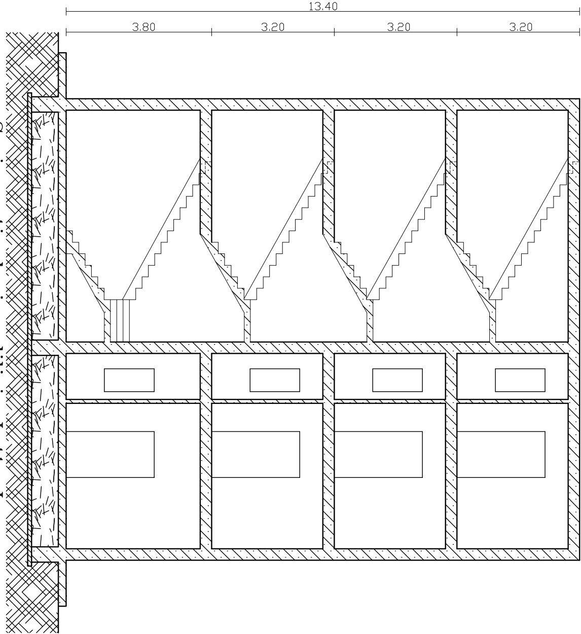
Sezione tipologia edilizia Lotto I
